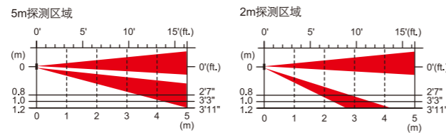
侧视图
