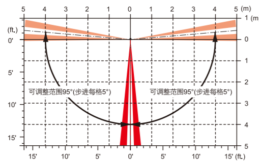
俯视图
